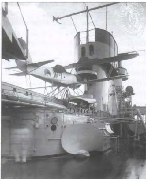
Vliegtuig aan boord H.M. De Ruyter. (Foto: Collectie S.J. Rosman.)
